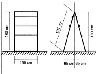
Šikmá stena
