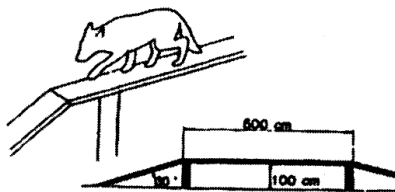
Obrázok č.12 Kladina nízka Používa sa na skúškach nižších typov. Umiestnená je vo výške jedného metra nad zemou, dlhá je 5 metrov a široká 30 centimetrov. Na začiatku a konci kladiny sú nábehové dosky so sklonom cca 30 stupňov.
