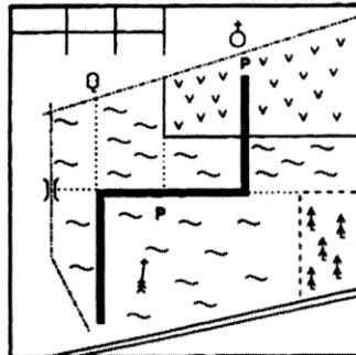
Obrázok č.3 Plánik stopy trasa stopy P predmet myslená priamka k záchytnému bodu cesta poľná cesta smer vetra mostík oranisko lúka ihličnatý les kostol ojedinelý listnatý strom
